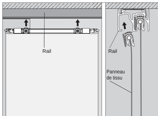
Pose et dépose faciles, directement par le bas, du chariot de guidage dans le rail
